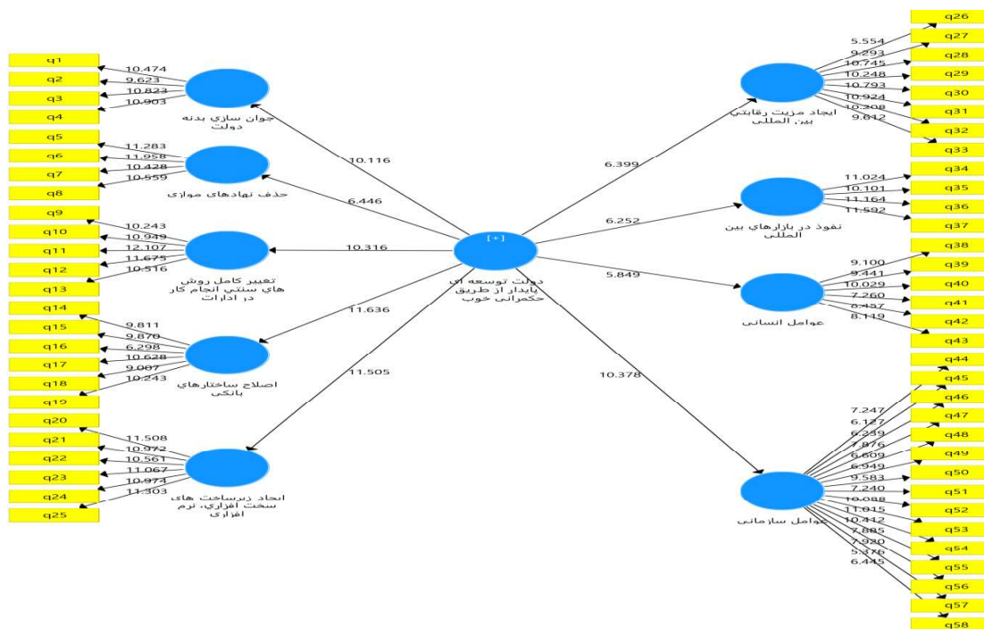
شکل ۵. مدل مفهومی پژوهش همراه با مقادیر t-value
